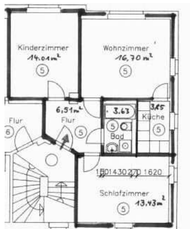
Grundriss
